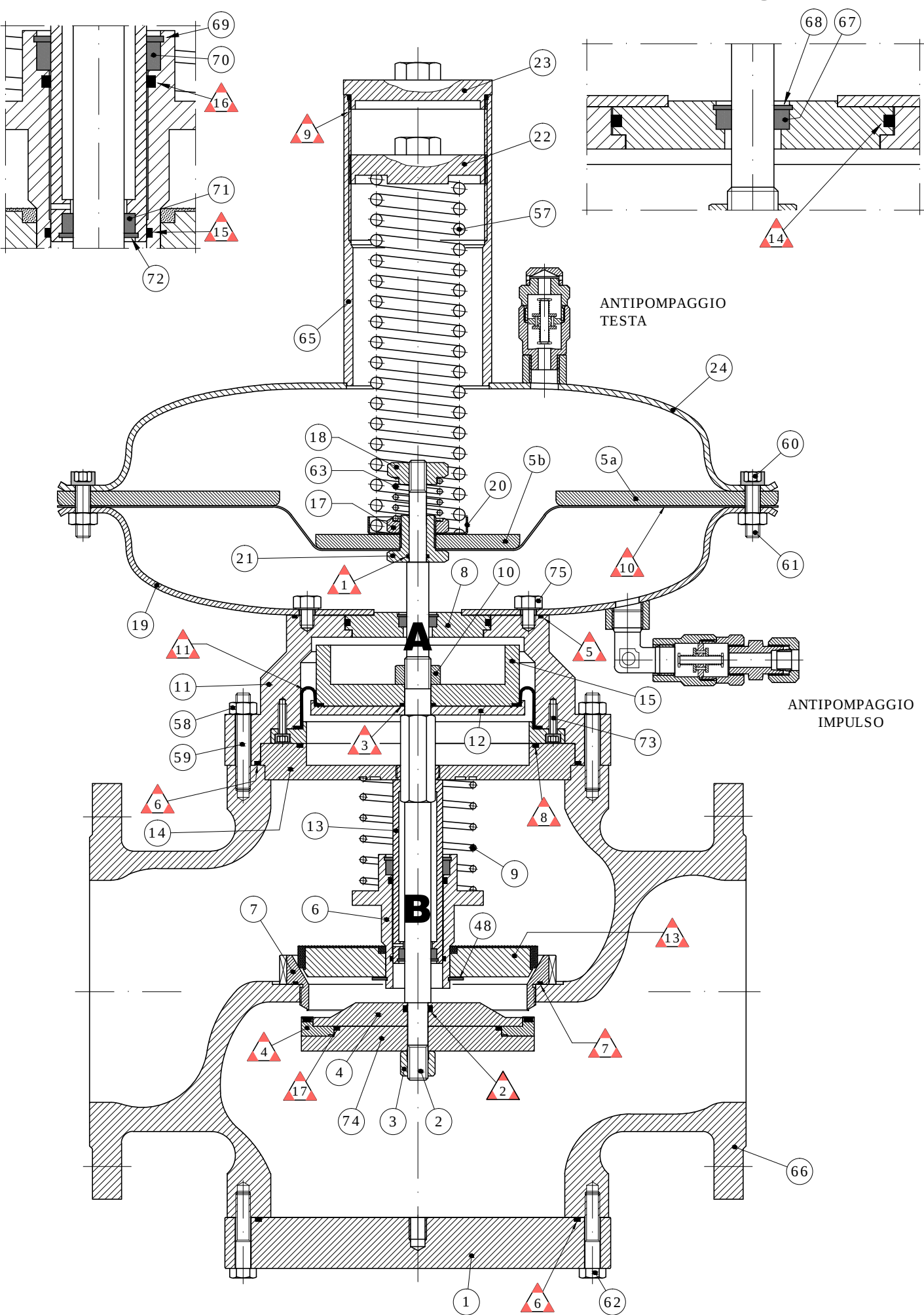
Dettaglio B
